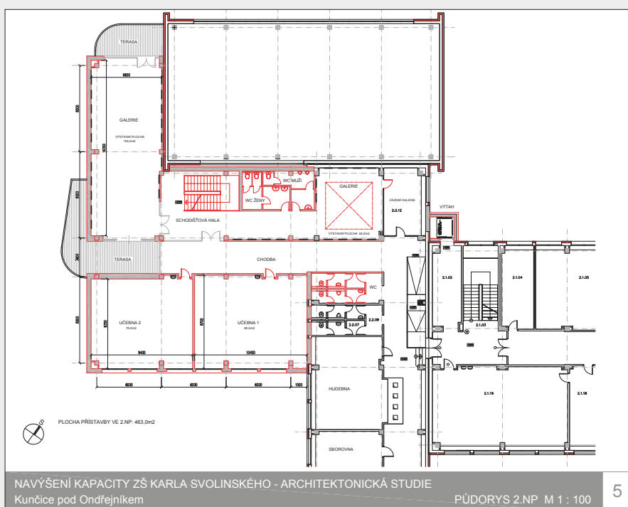
NAVÝŠENÍ KAPACITY ZŠ KARLA SVOLINSKÉHO - ARCHITEKTONICKÁ STUDIE Kunčice pod Ondřejníkem
